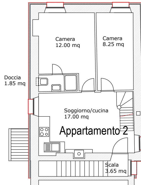
_secondo piano
