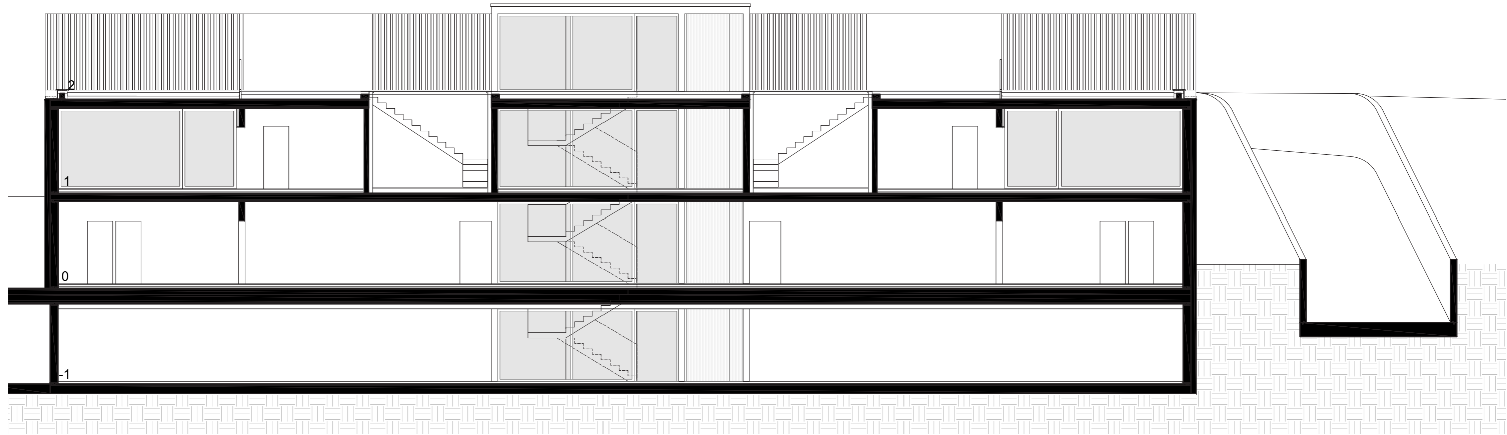
SEZIONE D-D
