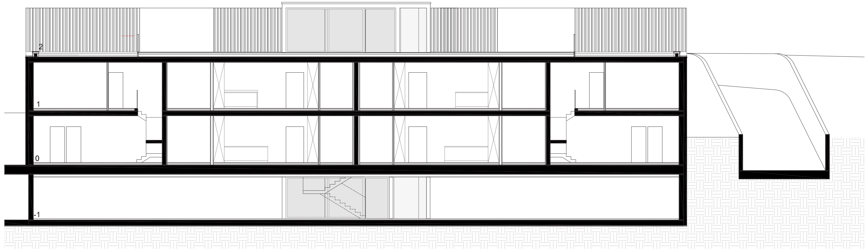
SEZIONE E-E
